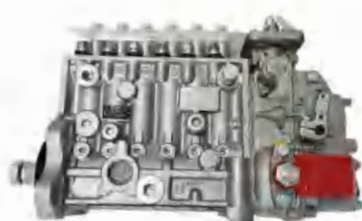
■ 6D114-2 ■ 6743-71-1131
