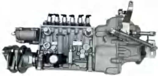
■ 6D170-2 ■ 6162-75-2160
