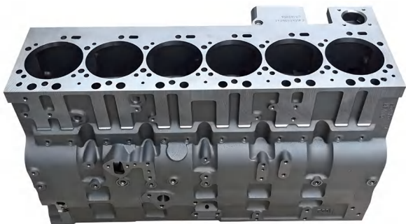
■ 6D114-3 ■ 6745-21-1190
